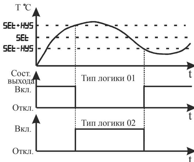
Рисунок 1 - Графическое представление типов логики работы выхода
