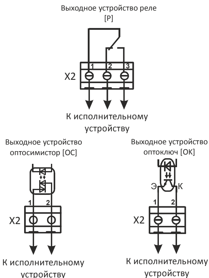
Рисунок 2 – Схемы подключения различных выходных устройств
