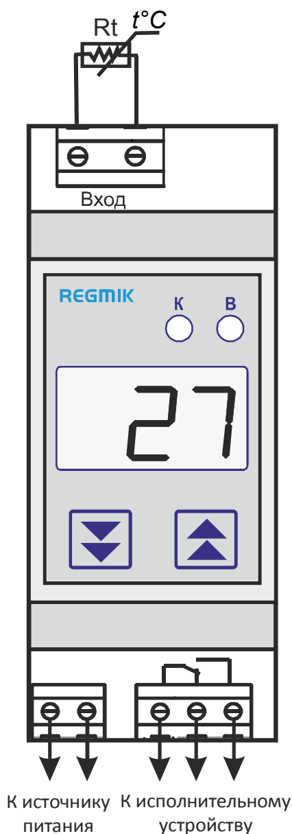
Рисунок 1 – Схема подключения прибора
